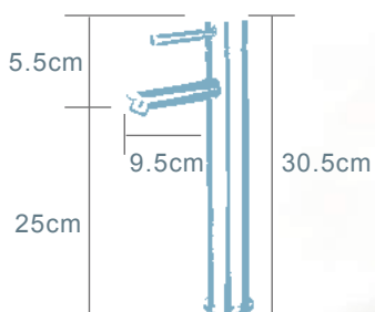
竹節單孔加高龍頭
