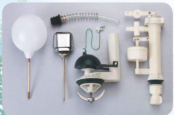
單體馬桶另件
